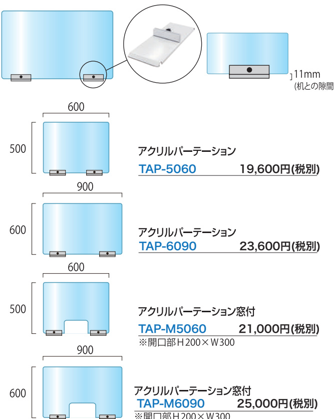
●アクリル板(透明)=厚さ3mm(※サイズにより異なります) ●ベース部=材質:スチール鋼板(SPHC) 表面処理:焼付け塗装(白色)
