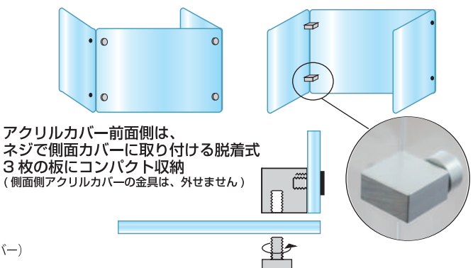
●アクリル板(透明)=厚さ3mm(※サイズにより異なります) ●金具=アルミ押し出し/B2アルマイト仕上(シルバー)
